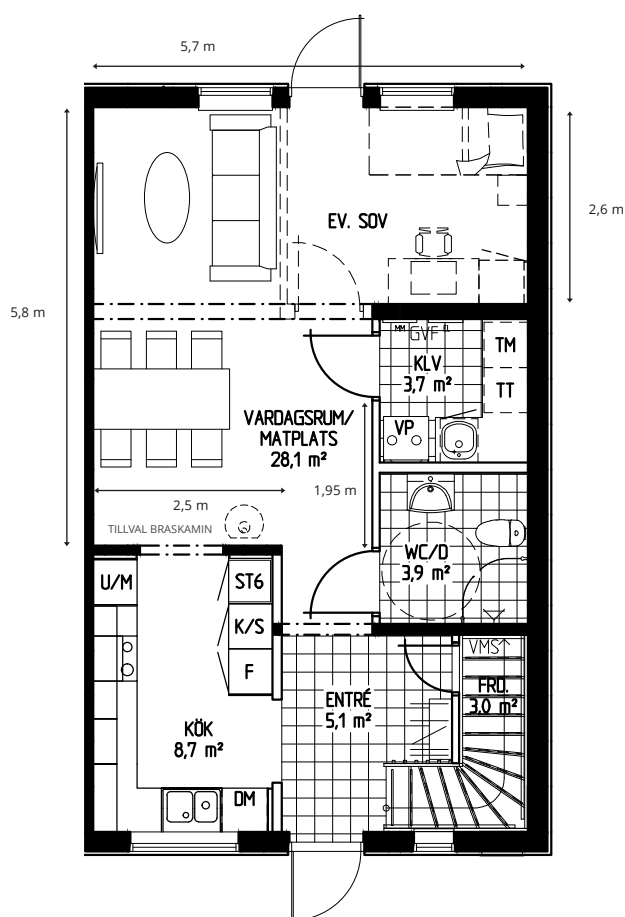
Undervåning
