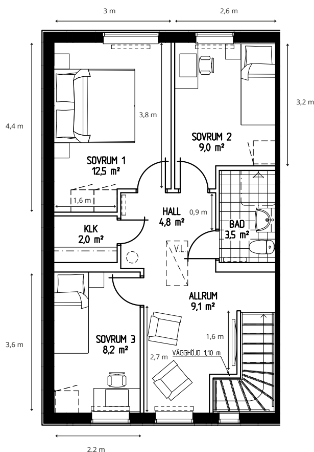
Övervåning
