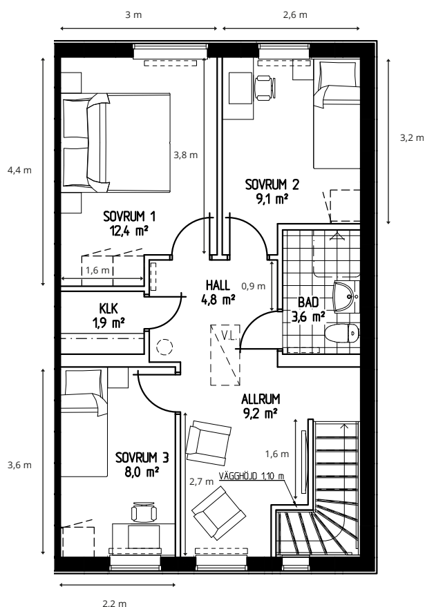
Övervåning
