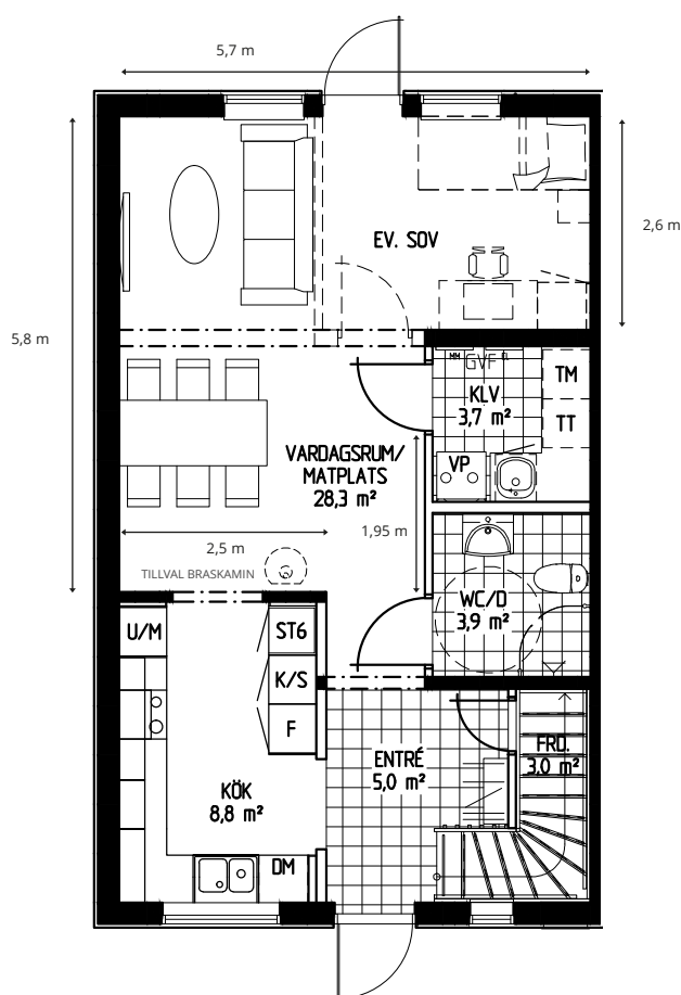
Undervåning
