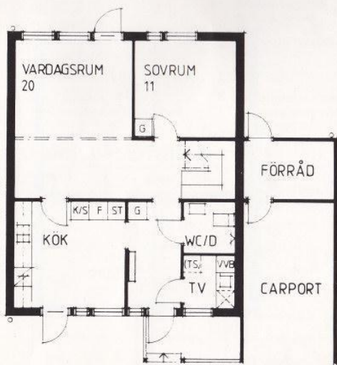
Bottenvåning
